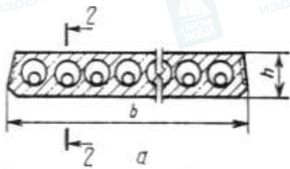
Плиты типов 1ПКТ, 2ПКТ, 3ПКТ
