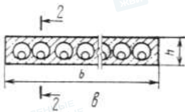
Плиты типов 1ПКК, 2ПКК, 3ПКК
