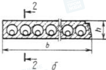
Плиты типов 1ПКТ, 2ПКТ, 3ПКТ
